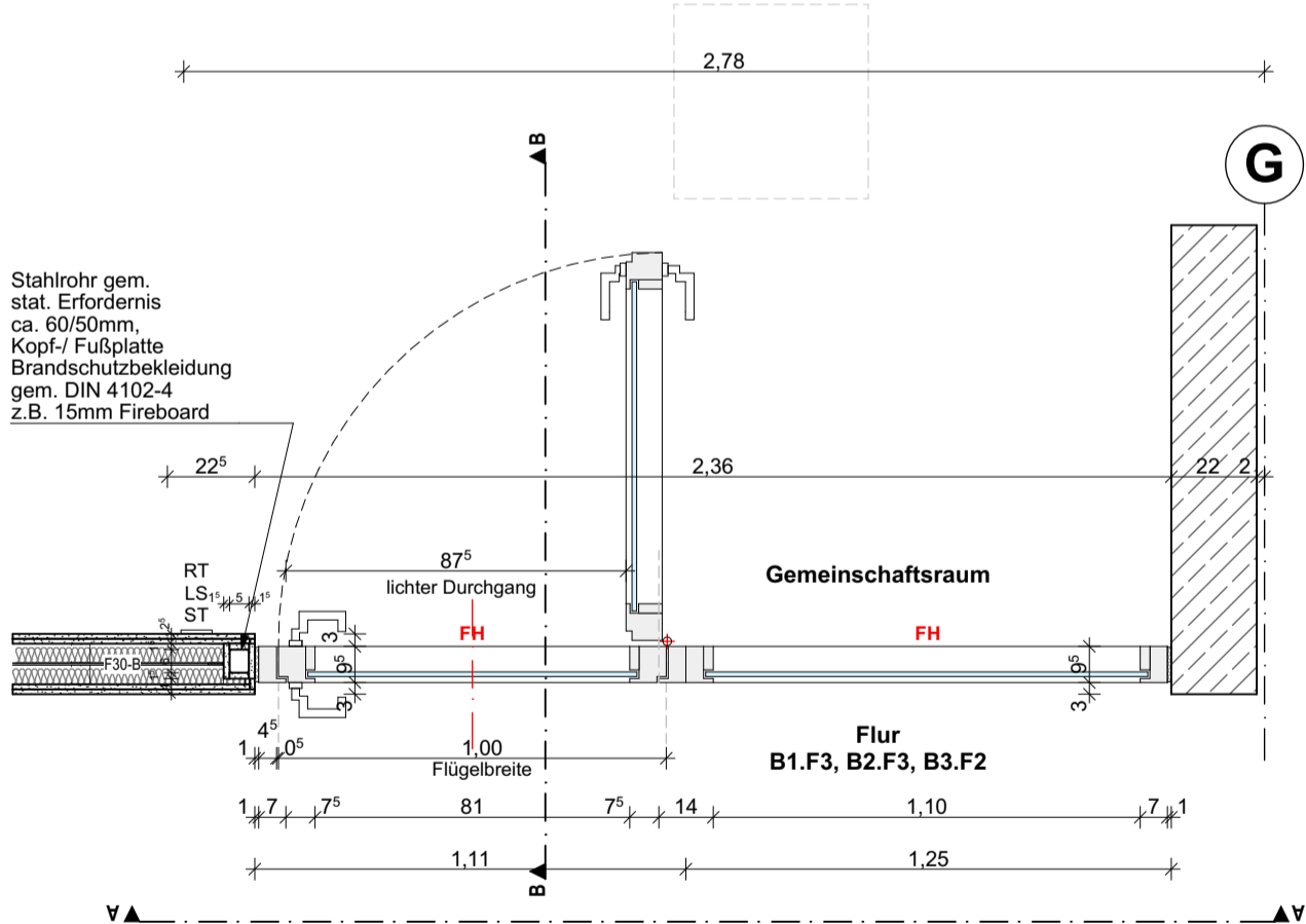
Grundriss
