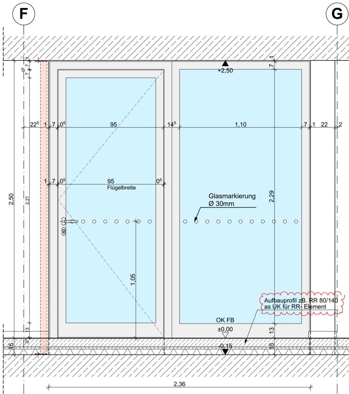
Schnittansicht A - A
